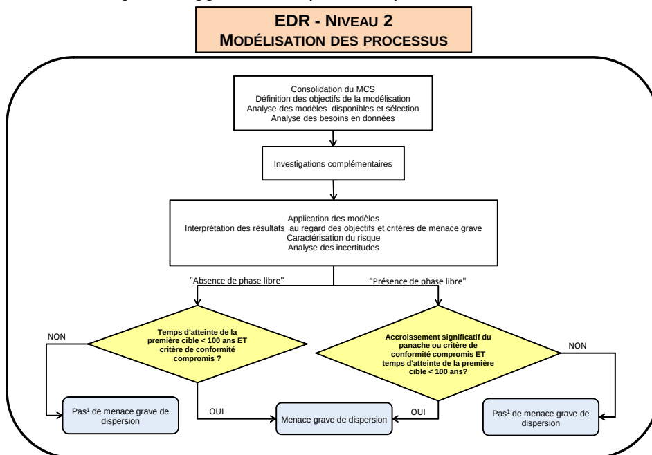
Figure 10 – Logigramme détaillé pour l'EDR dispersion – Niveau 2
