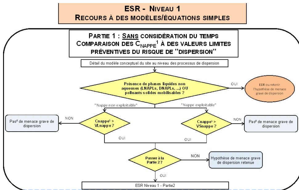
Figure 8 –Logigramme détaillé pour l'ESR-N dispersion - Partie 1
