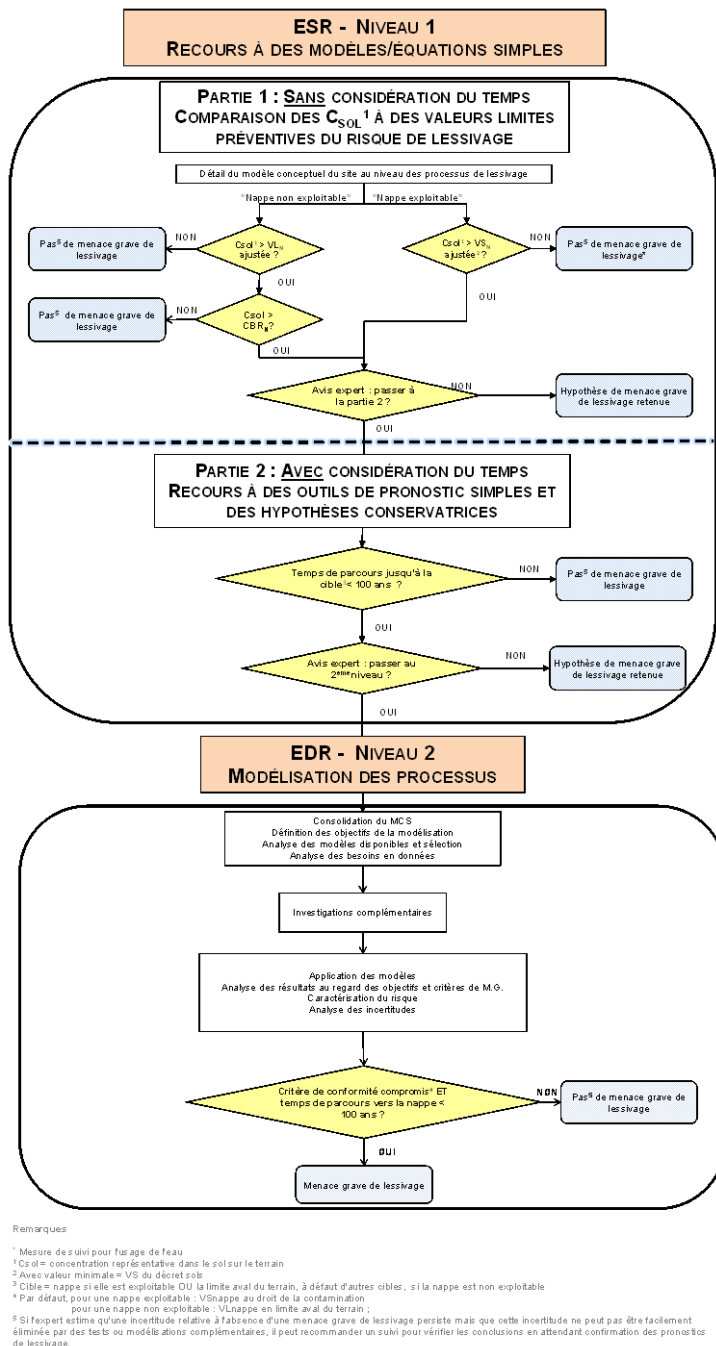
Figure 3- Logigramme méthodologique général pour le module lessivage
