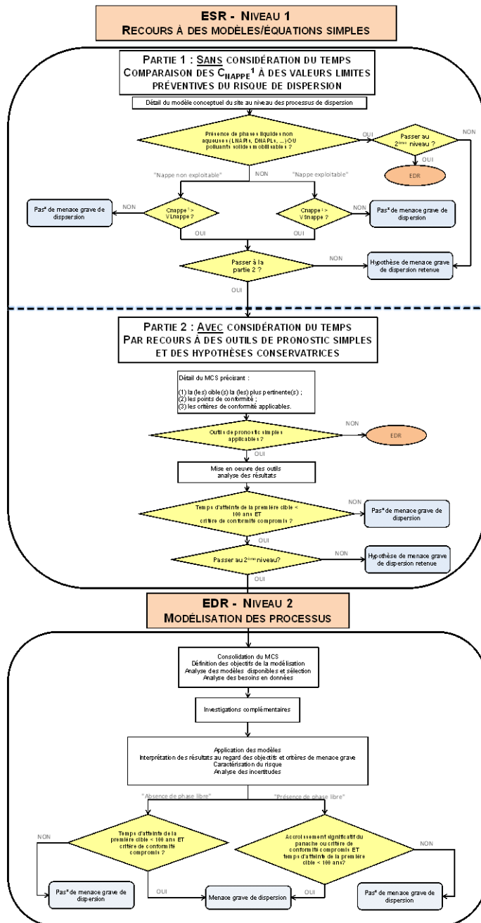
Figure 4 – Logigramme méthodologique pour le module dispersion
