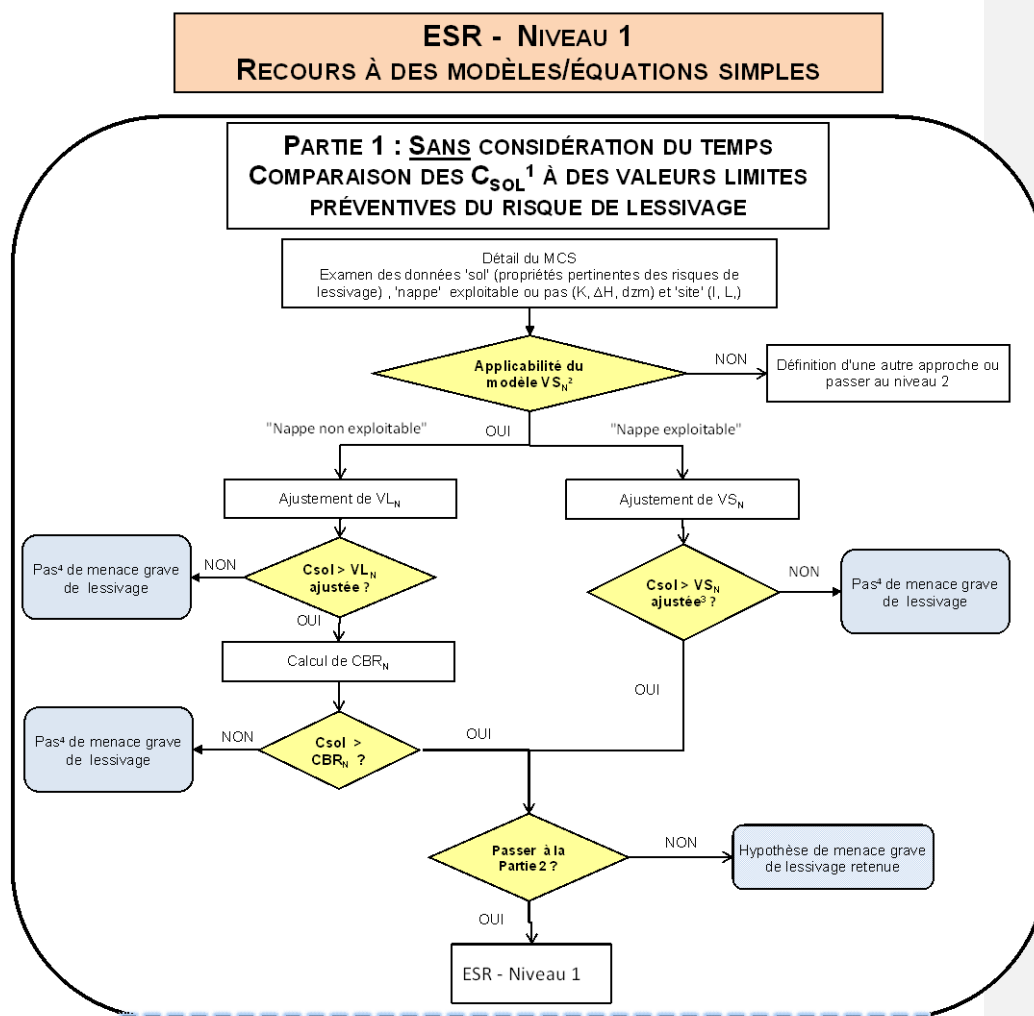
Figure 5 – Logigramme détaillé pour l'ESR lessivage - Niveau 1 sans considération du temps
