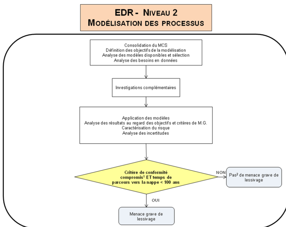
Figure 7 – Logigramme détaillé pour l'EDR lessivage
