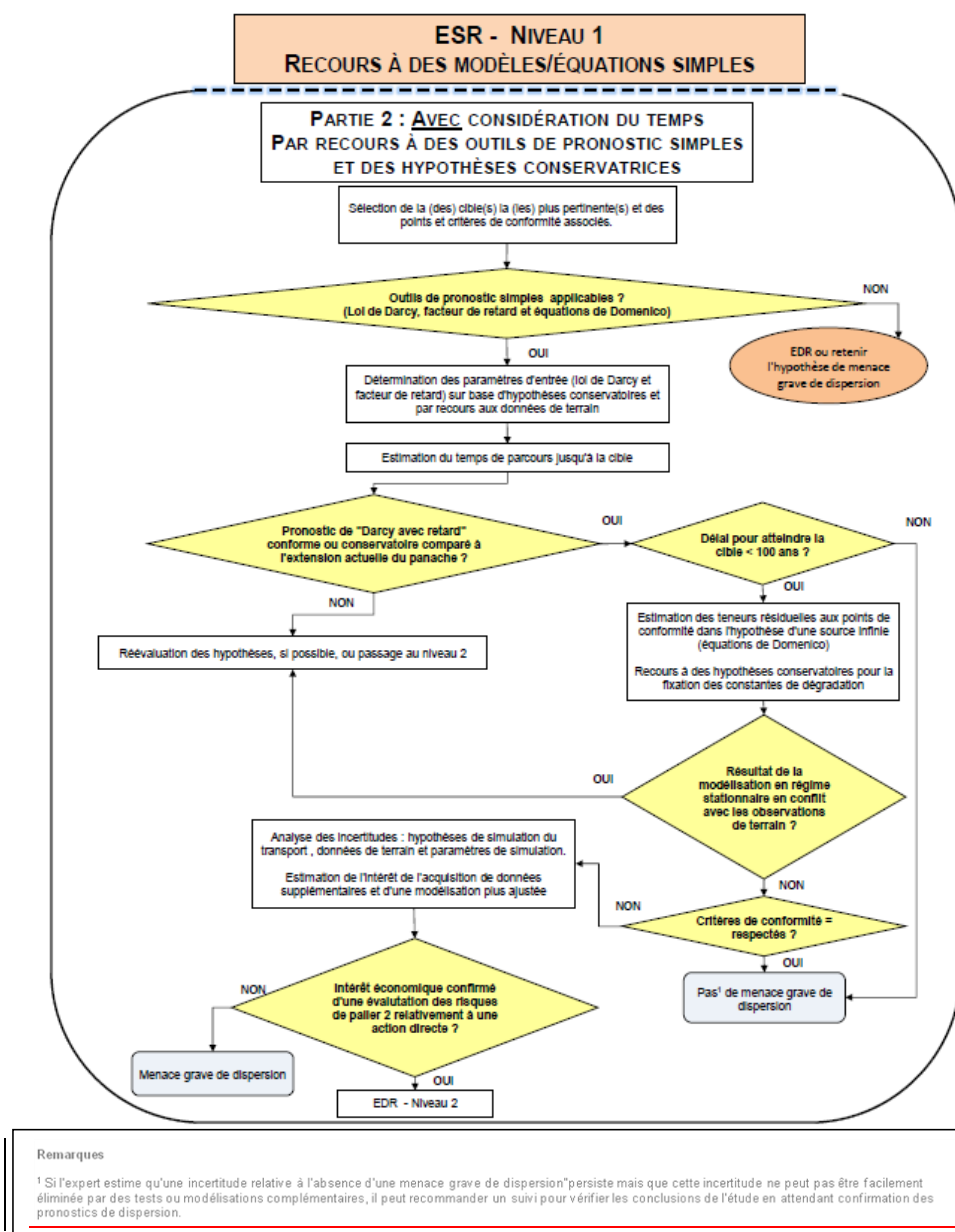
Figure 9 – Logigramme détaillé pour l'ESR –N dispersion Partie 2 par recours à des outils de pronostic simples et des hypothèses conservatoires
